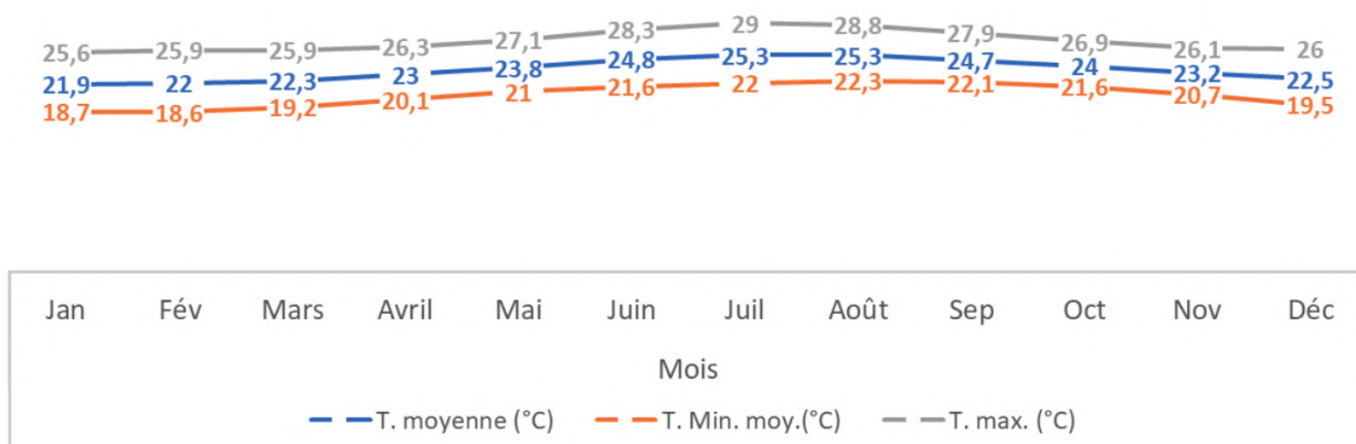
FIGURE 6: GRAPHE DES TEMPÉRATURES DE LA COMMUNE DE GRAND GOSIER, SOURCE : FR.CLIMATE-DATA.ORG
